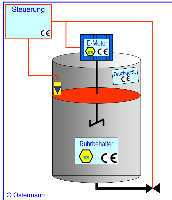
Rührgerät (Prinzipskizze)
